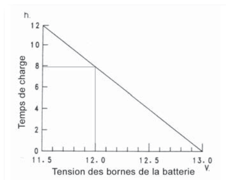
Graphique du temps de charge selon la tension en bornes.
